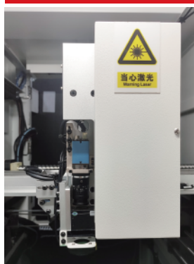
CO 2 激光头
